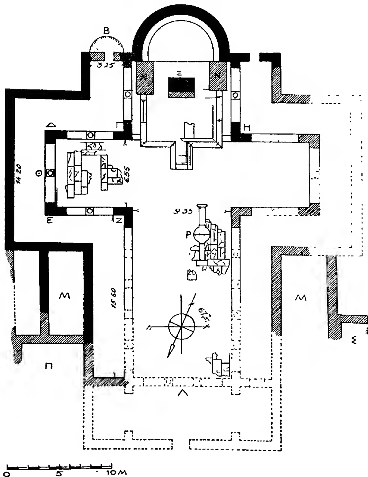
FIG. 1. — THASOS, BASILIQUE CRUCIFORME : PLAN d'après A. ORLANDOS.
